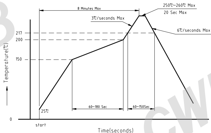
回流焊曲线图
